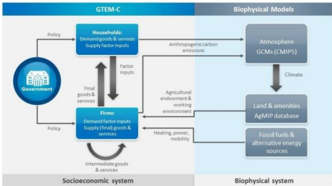
Figura 28: Estrutura do modelo GTEM-C
