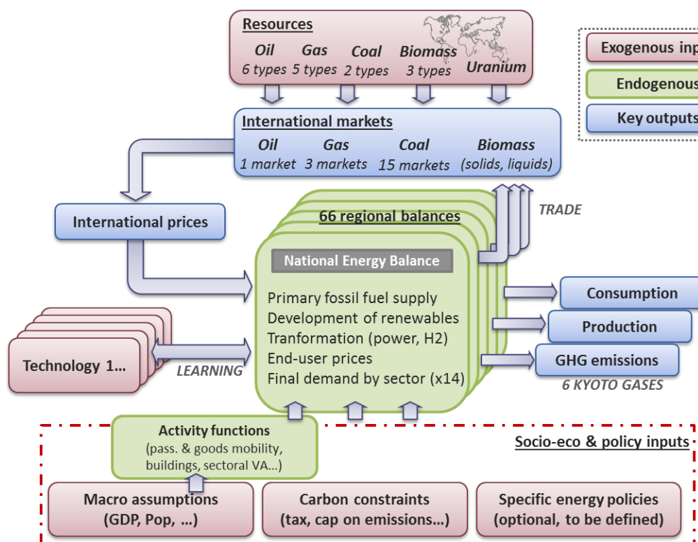
Figura 19: Estrutura do modelo POLES
