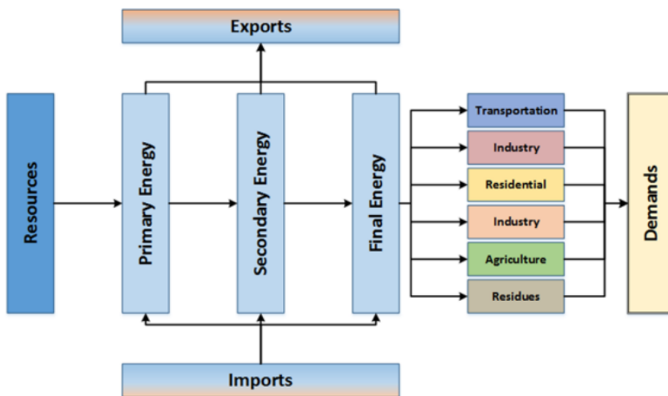
Figura 9: Representação do sistema energético do modelo COFFEE
