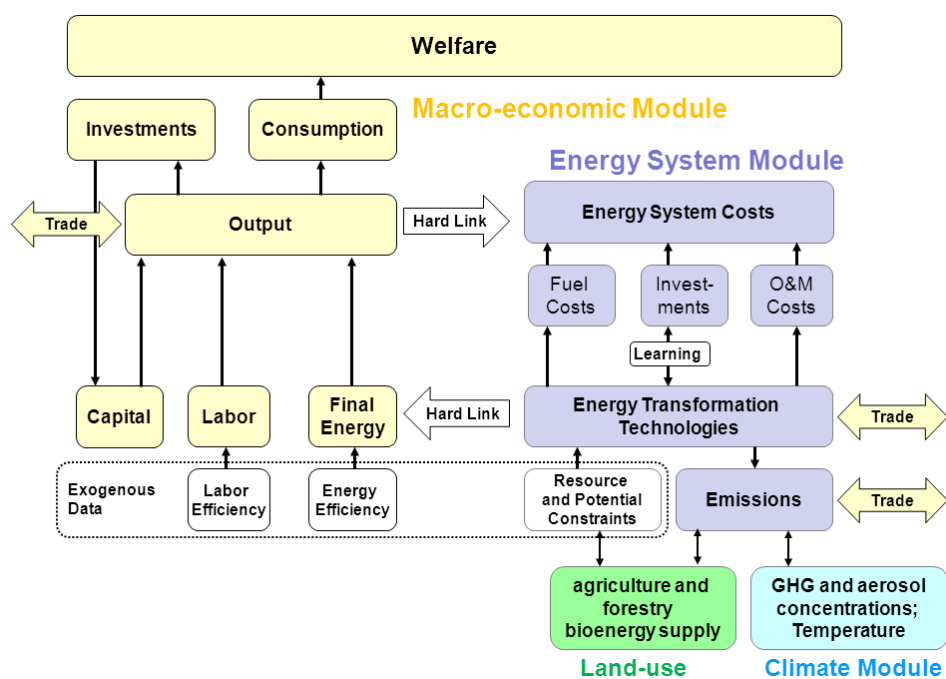
Figura 20: Estrutura geral do modelo REMIND
