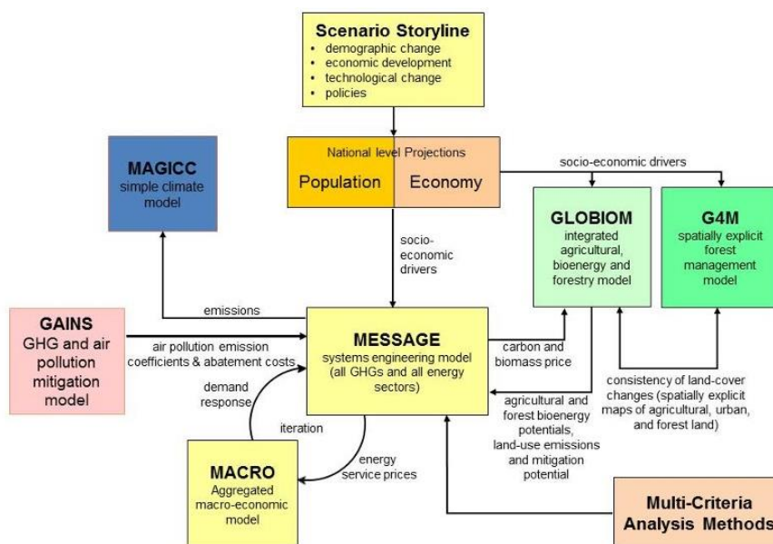
Figura 18: Visão geral da estrutura do modelo MESSAGE
