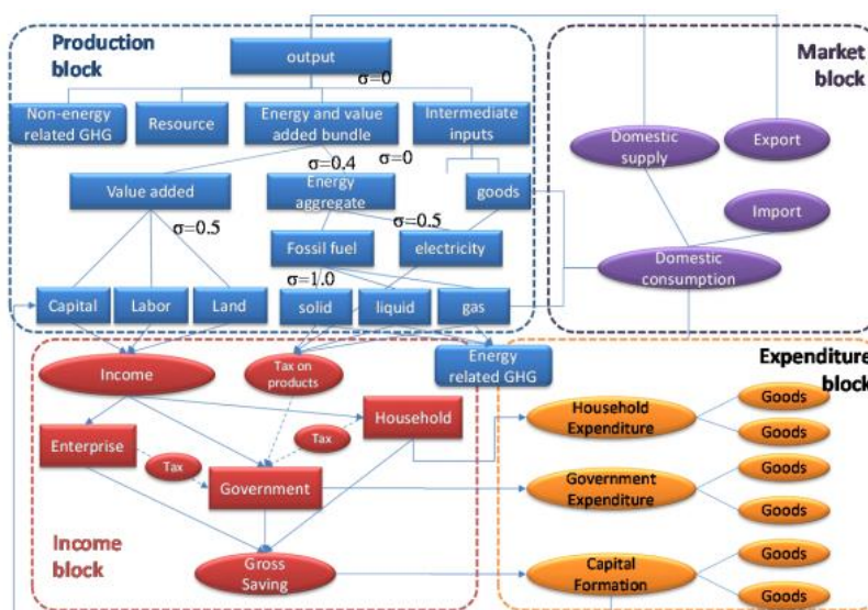
Figura 8: Visão geral da estrutura do modelo AIM/CGE
