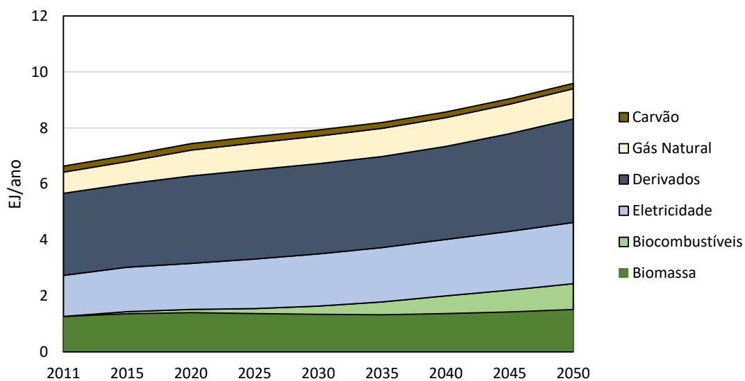
Figura 77: Consumo final de energia do Brasil no cenário REF do modelo TEA
