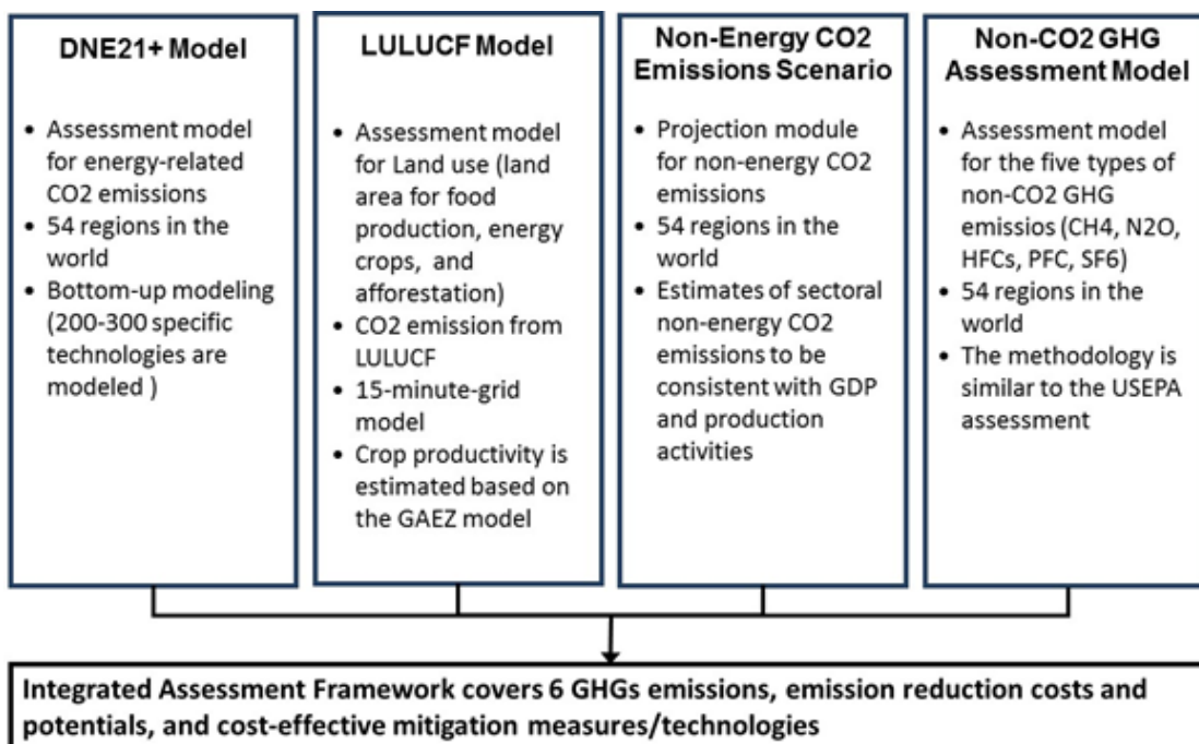
Figura 10: Estrutura do modelo DNE21+
