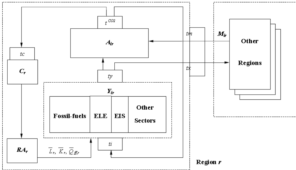
Figura 32: Estrutura esquemática do modelo PACE
