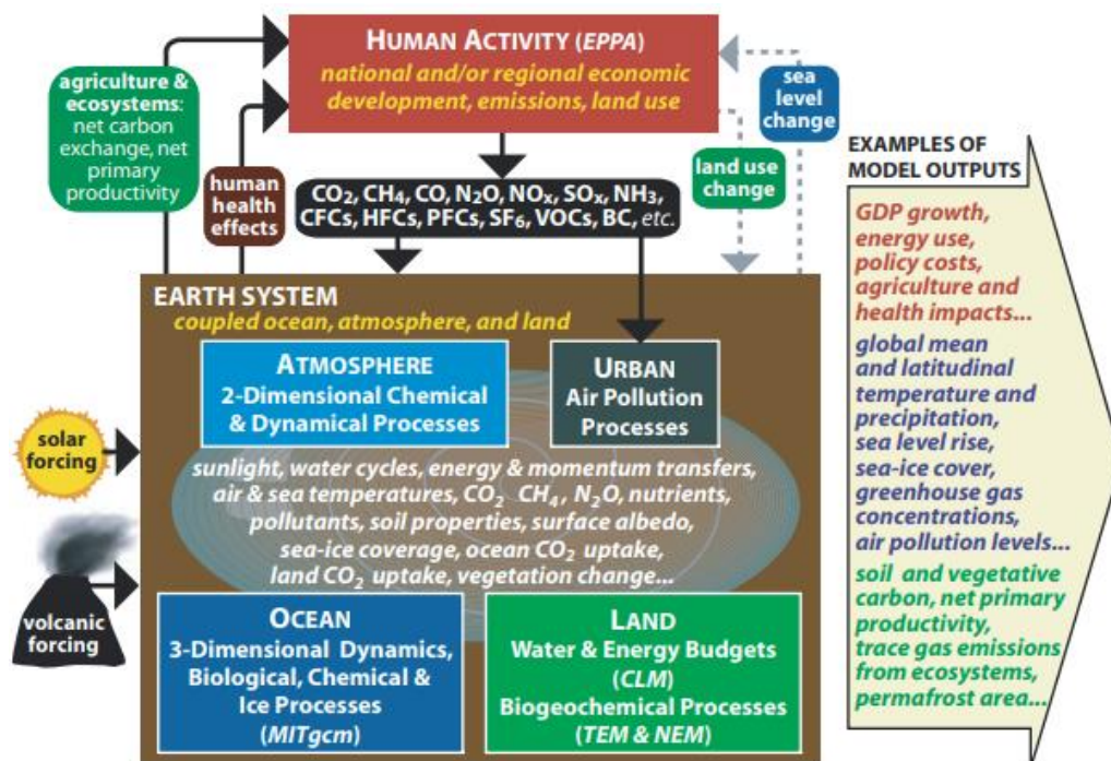
Figura 14: Esquema do funcionamento do modelo IGMS
