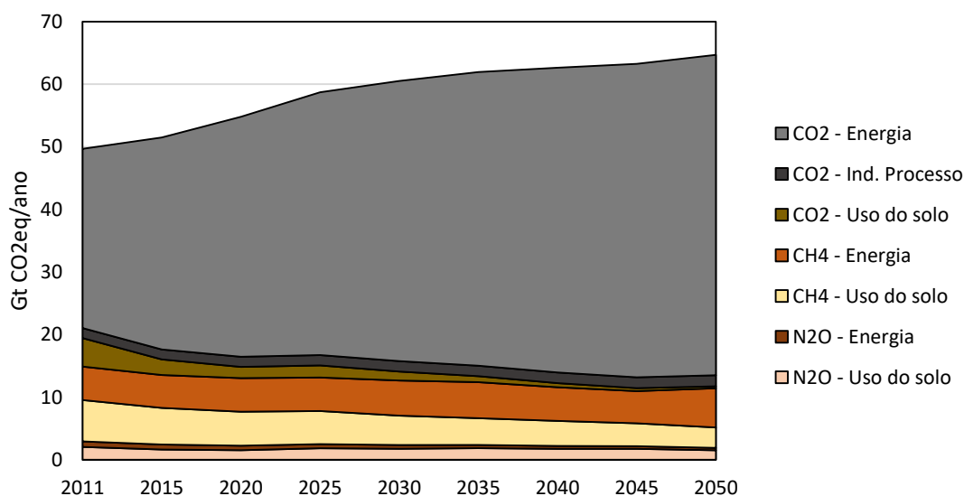
Figura 78: Emissões de GEE globais por tipo de gás e origem no cenário REF do modelo TEA
